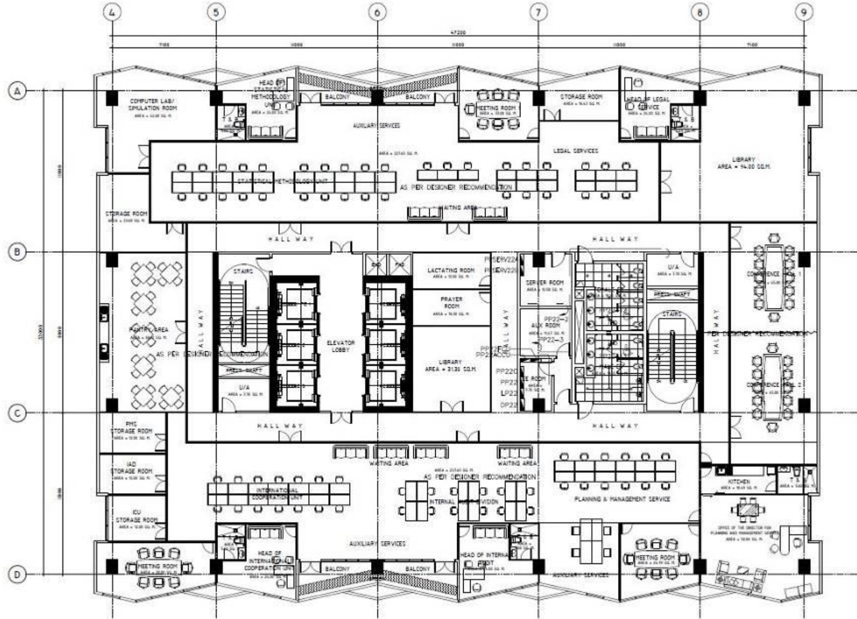
POWER LAYOUT SCALE: 1:200 MTS
